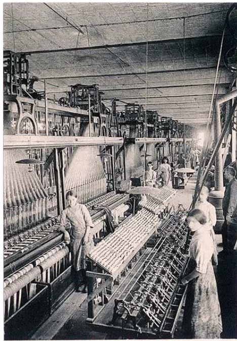
27 - GROBER y C.ª - Fábrica de Gerona. Telares mecánicos con Jacquard, para la fabricación de galones, agremanes, etc.
